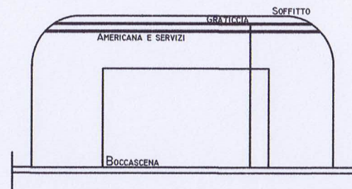
SEZIONE PALCOSCENICO
