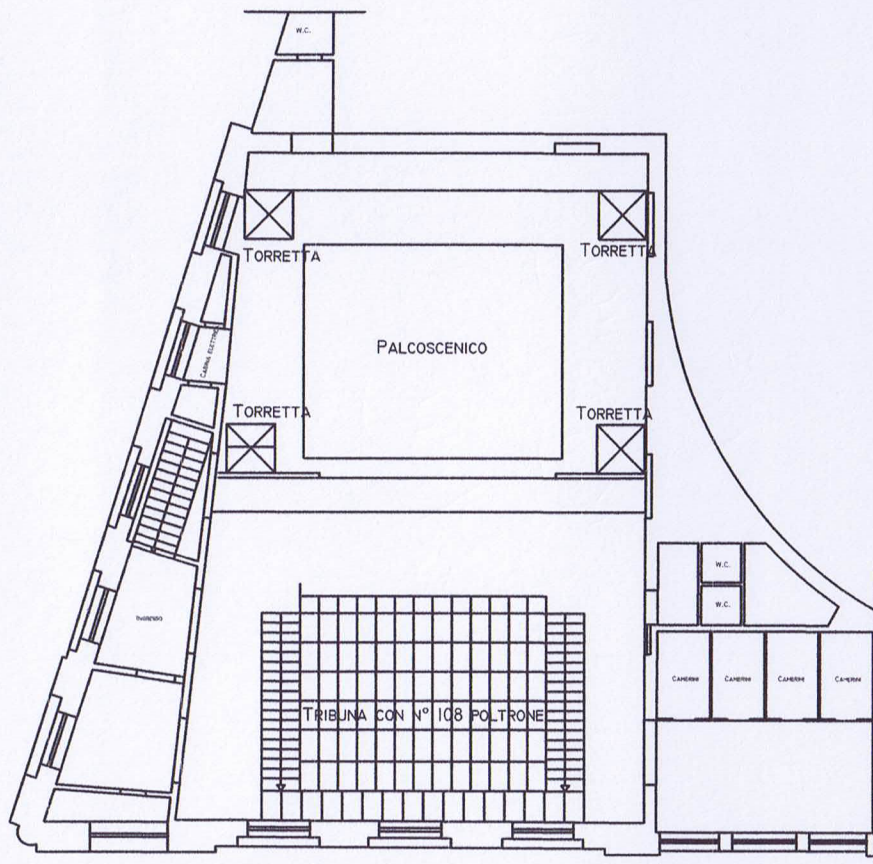
PLANIMETRIA PALCOSCENICO
