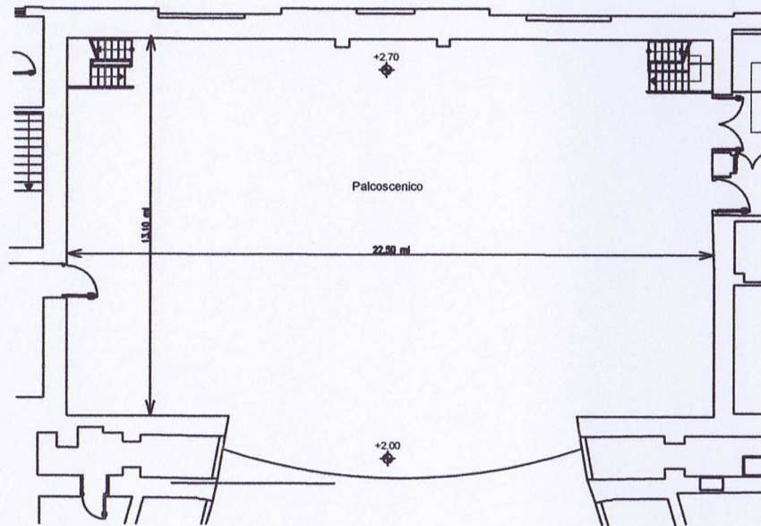
PLANIMETRIA PALCOSCENICO
