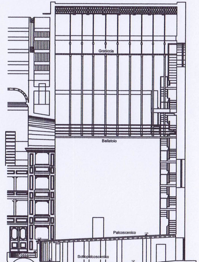
SEZIONE PALCOSCENICO
